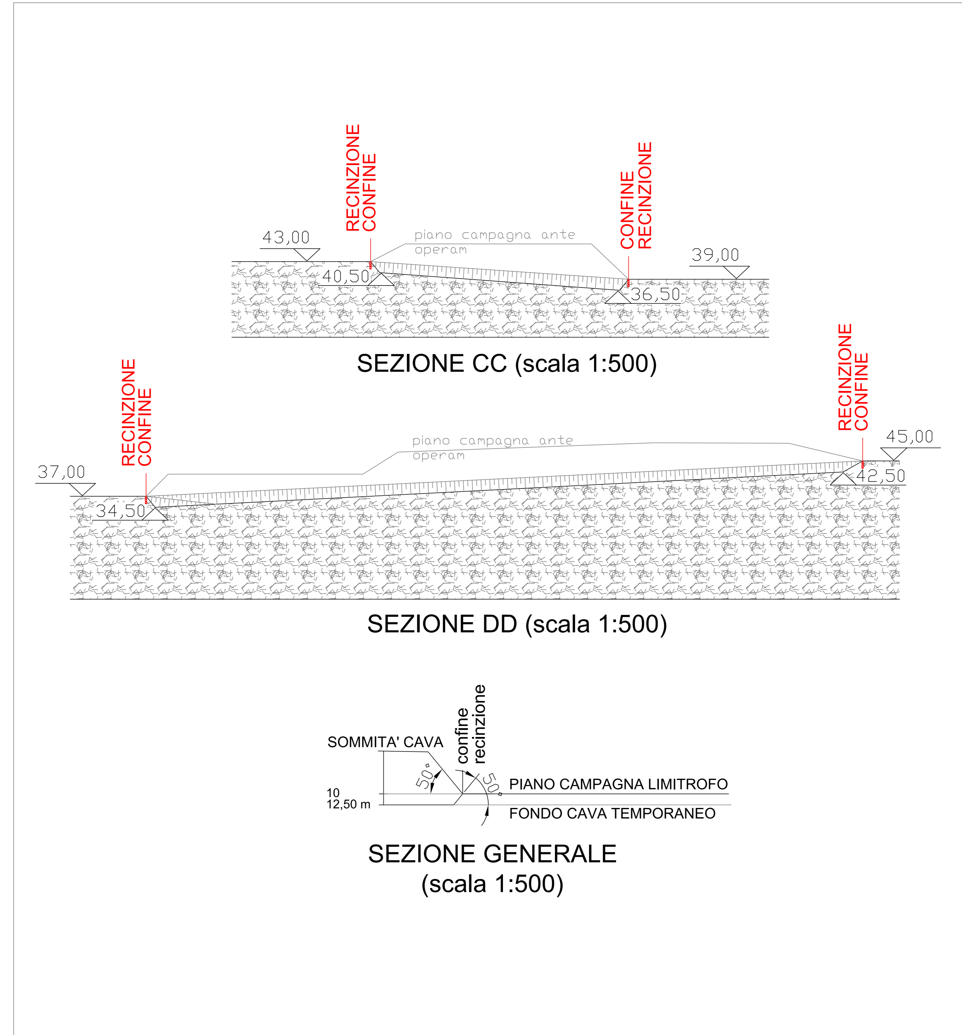
SEZIONI DI PROGETTO (scala 1:500)
