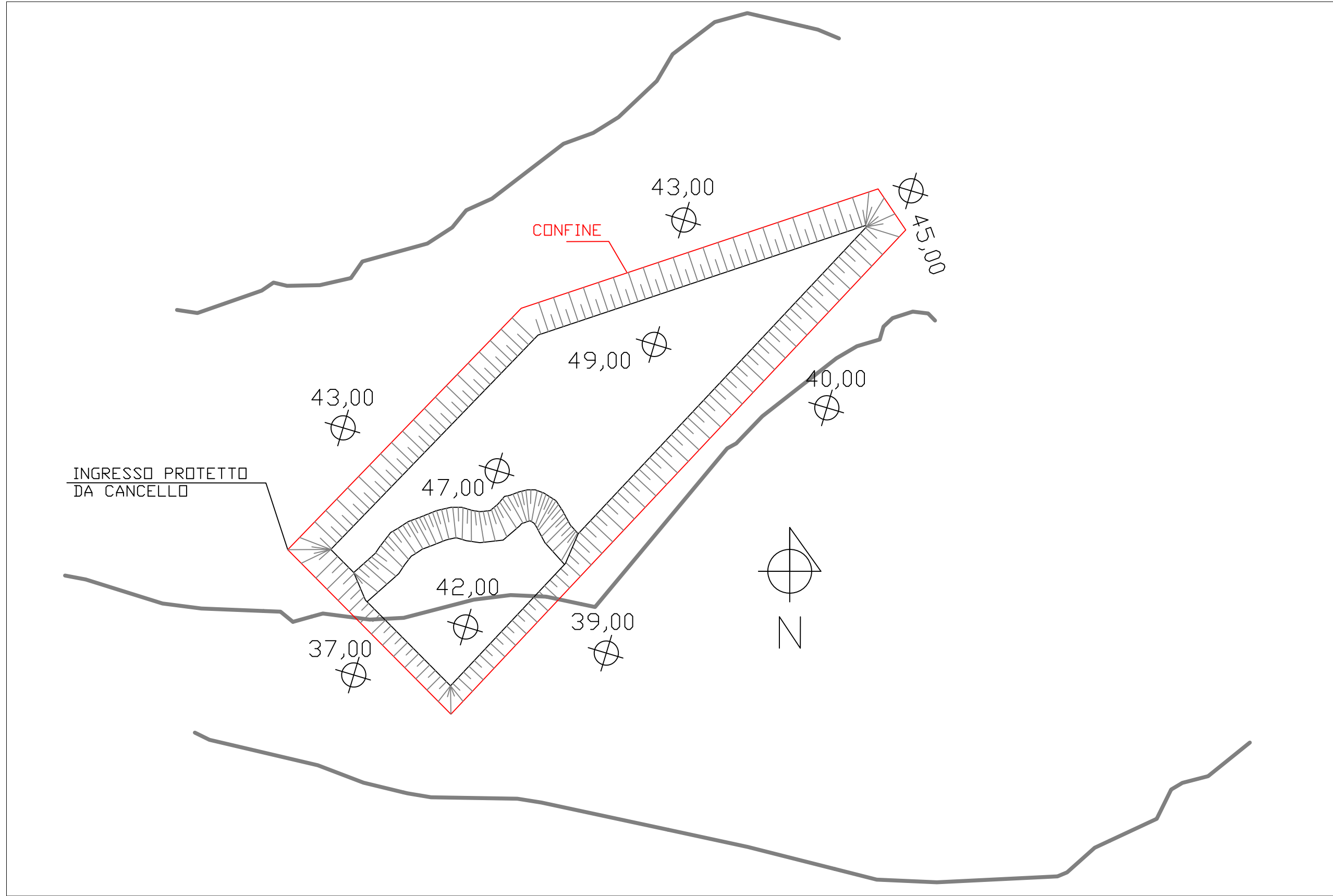
PLANIMETRIA (scala 1:1000)
