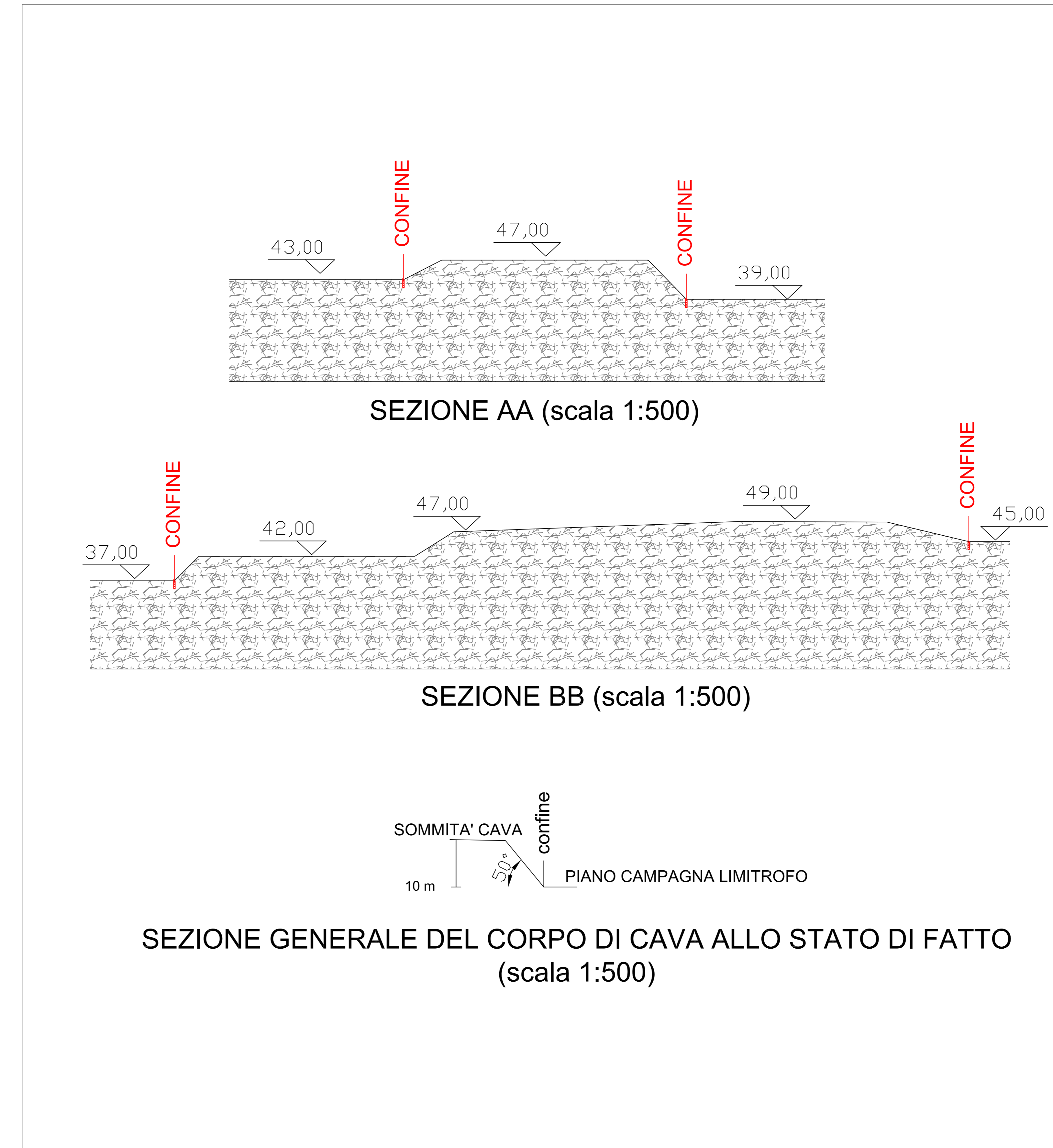
SEZIONI STATO DI FATTO (scala 1:500)
